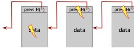
Eine als Kette von Datenblöcken („Blockchain“) strukturierte Datenbank
